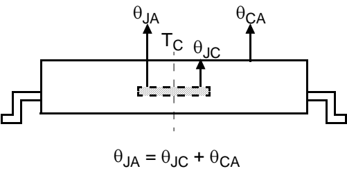
Figure 14. Thermal Resistance(°C/Watt)
